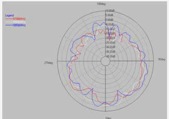
5G (PHI=90)
