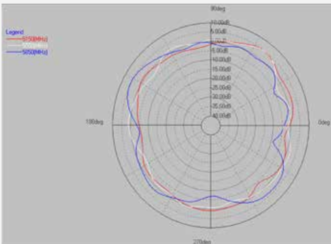
5G (PHI=0)
